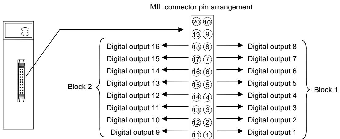
H-DO-D module
