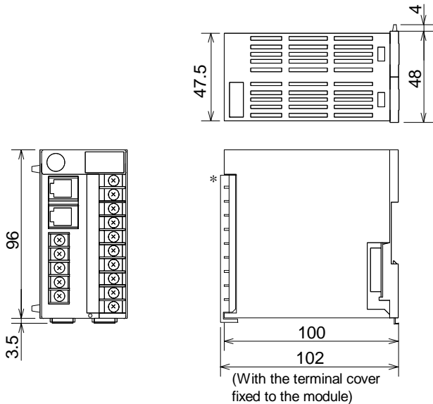
H-PCP module
