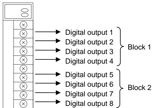
H-DO-A module
