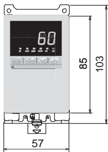
DIN rail mounting type
